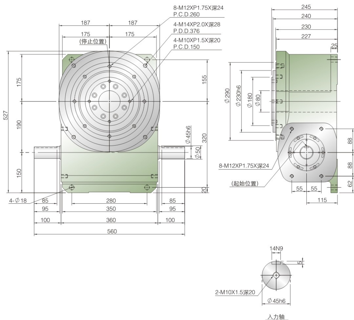
入力軸
