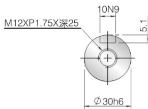
出力轴
