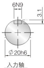
入力轴
